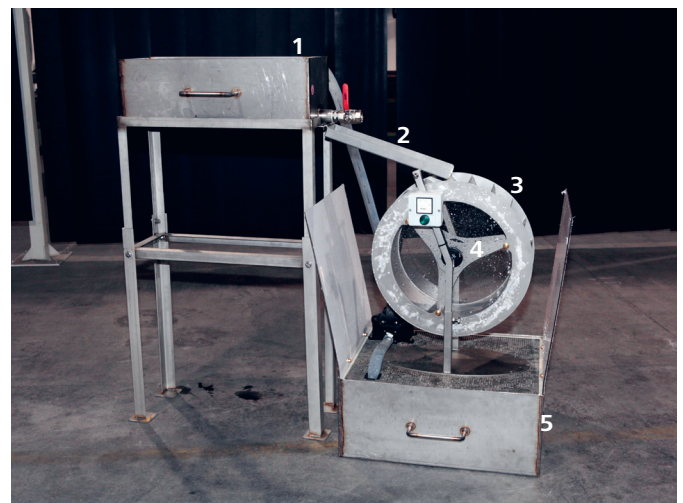
Das Wasserradmodell
